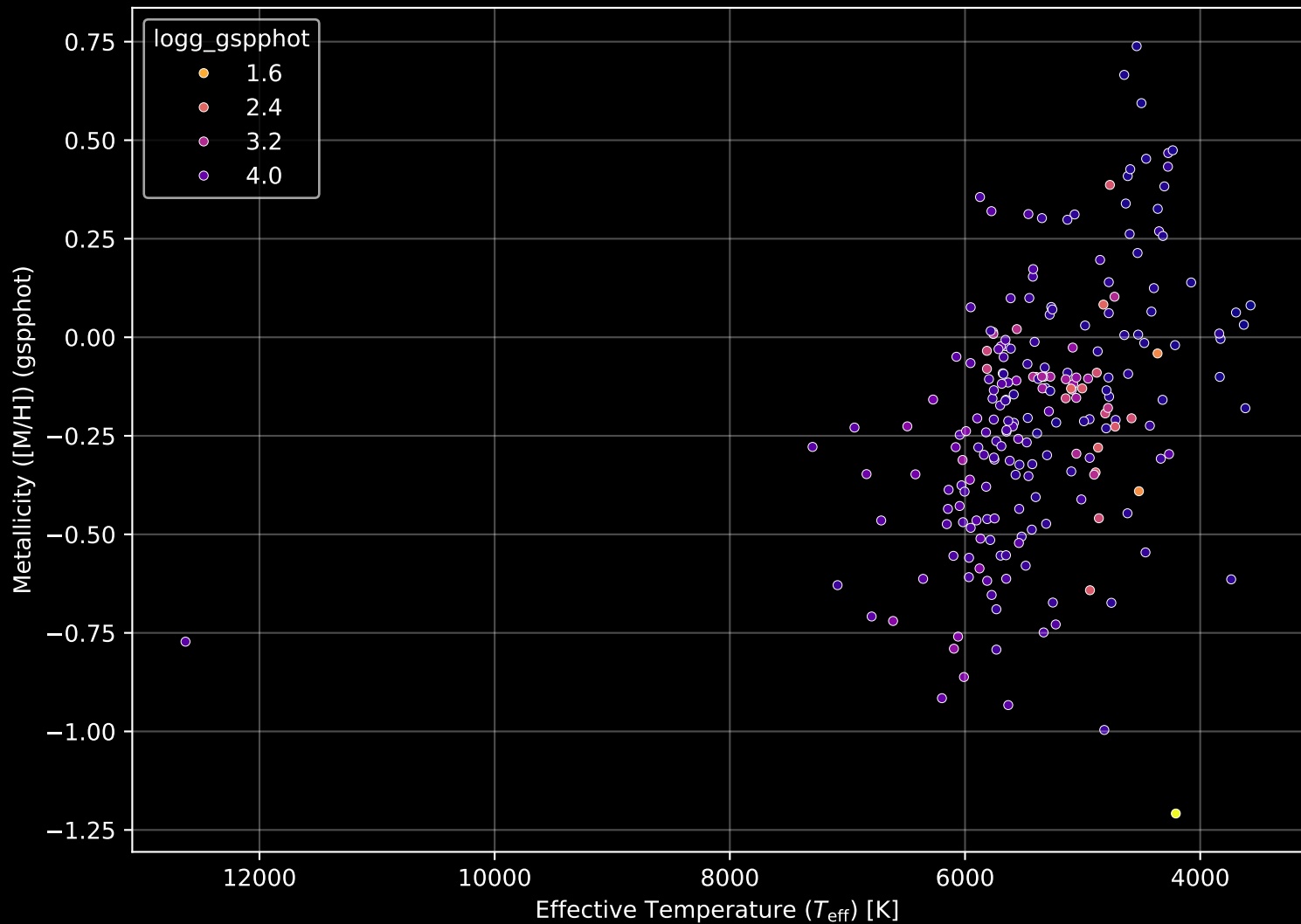
APOGEE DR17 Field: [160-60] Stellar Population Parameters (n= 219)
